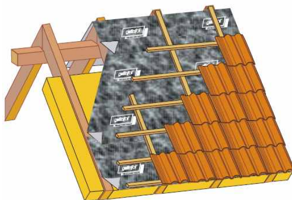
Schéma položení folie GUTTAFOL DO 95
