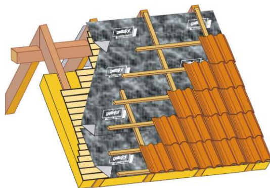
Schéma položení fólie EUROFOL
